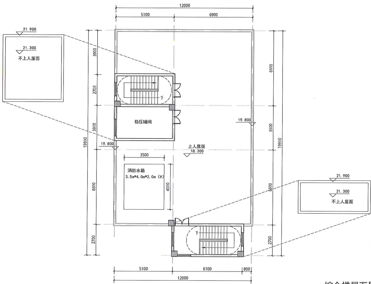
综合楼屋面层平面图
