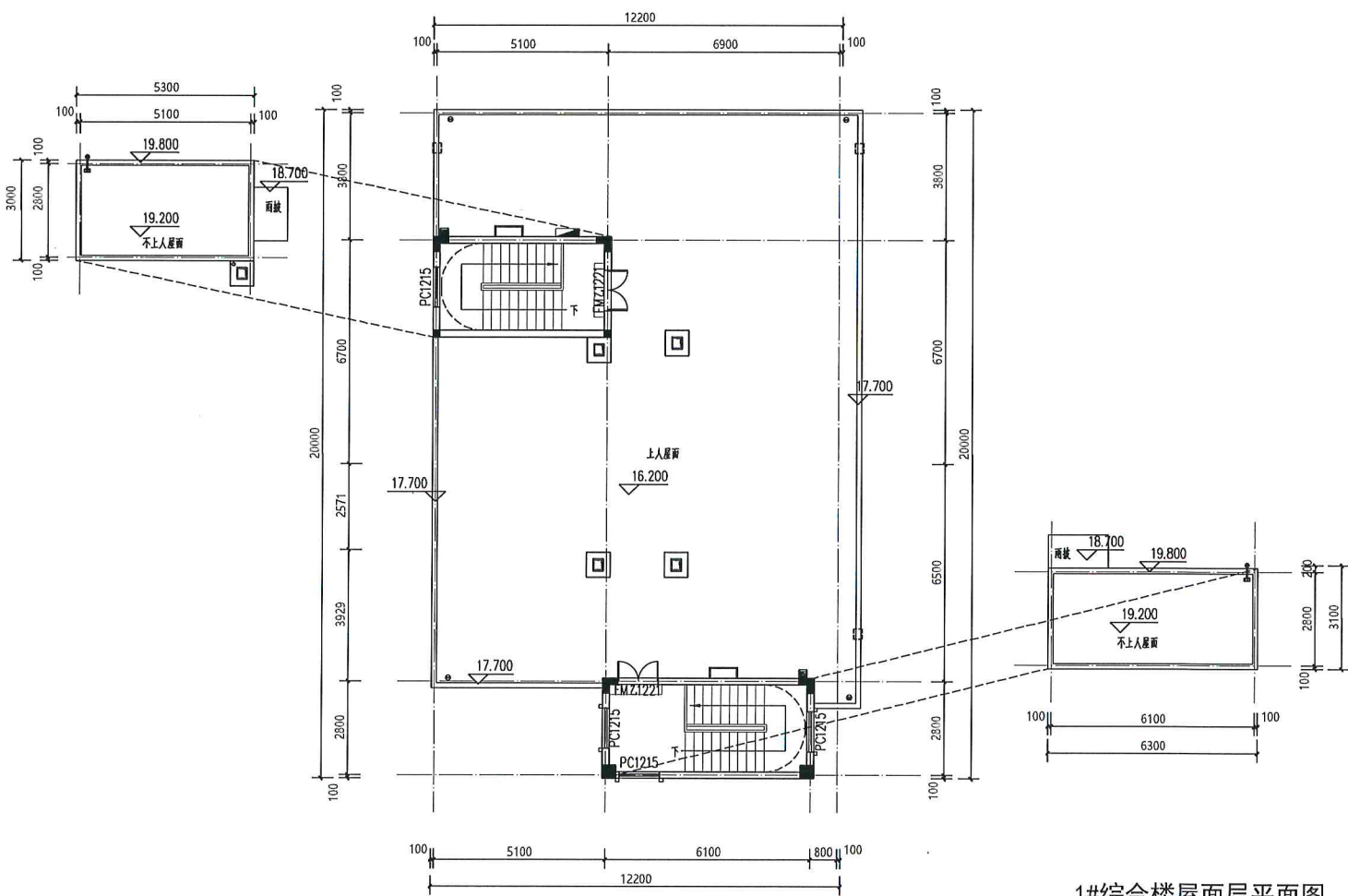
1#综合楼屋面层平面图
