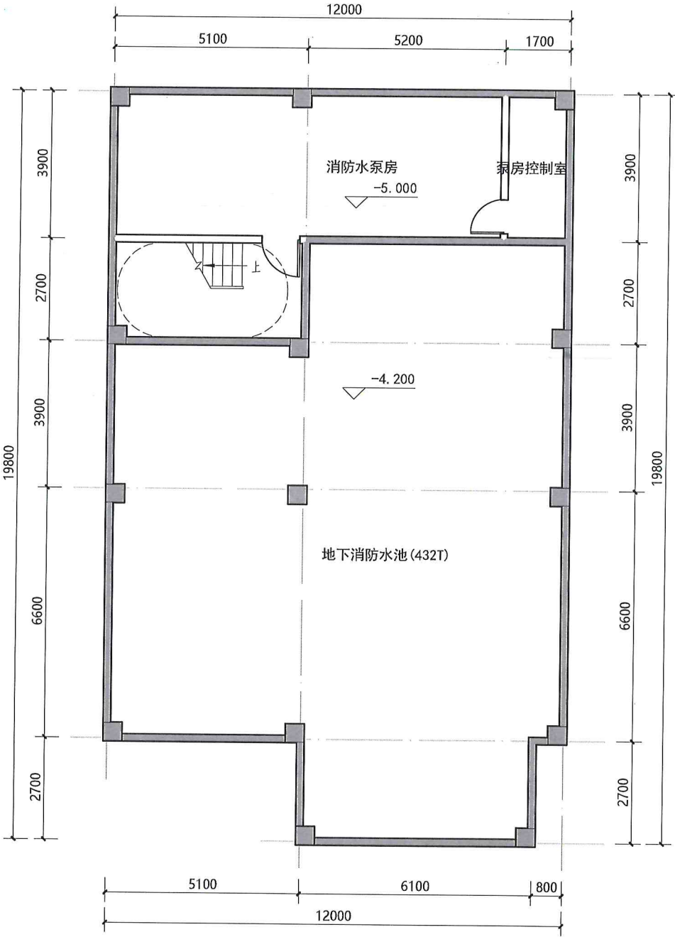
1#综合楼地下一层平面图
