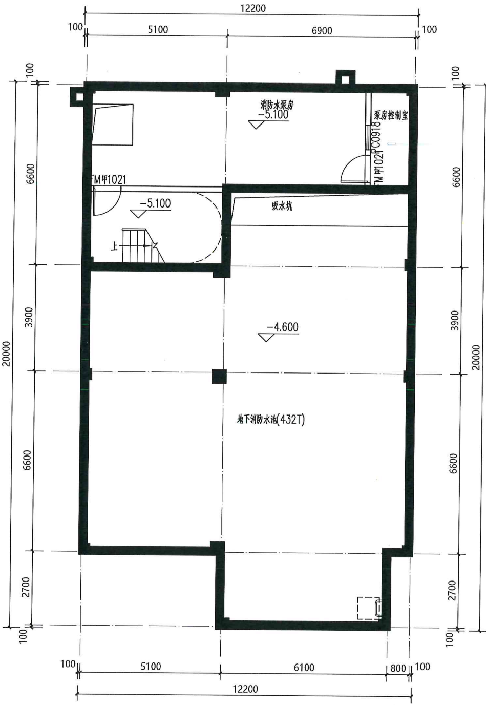
1#综合楼地下一层平面图
