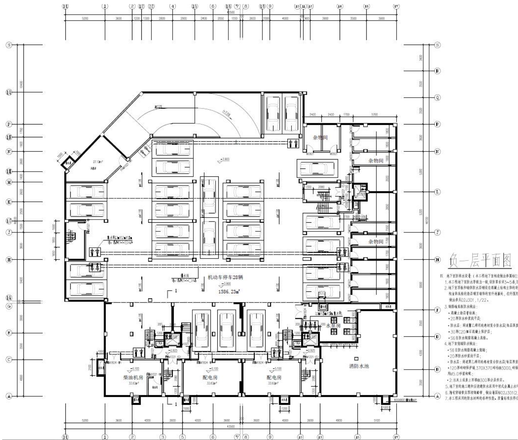
负一层平面图 (变更前)
