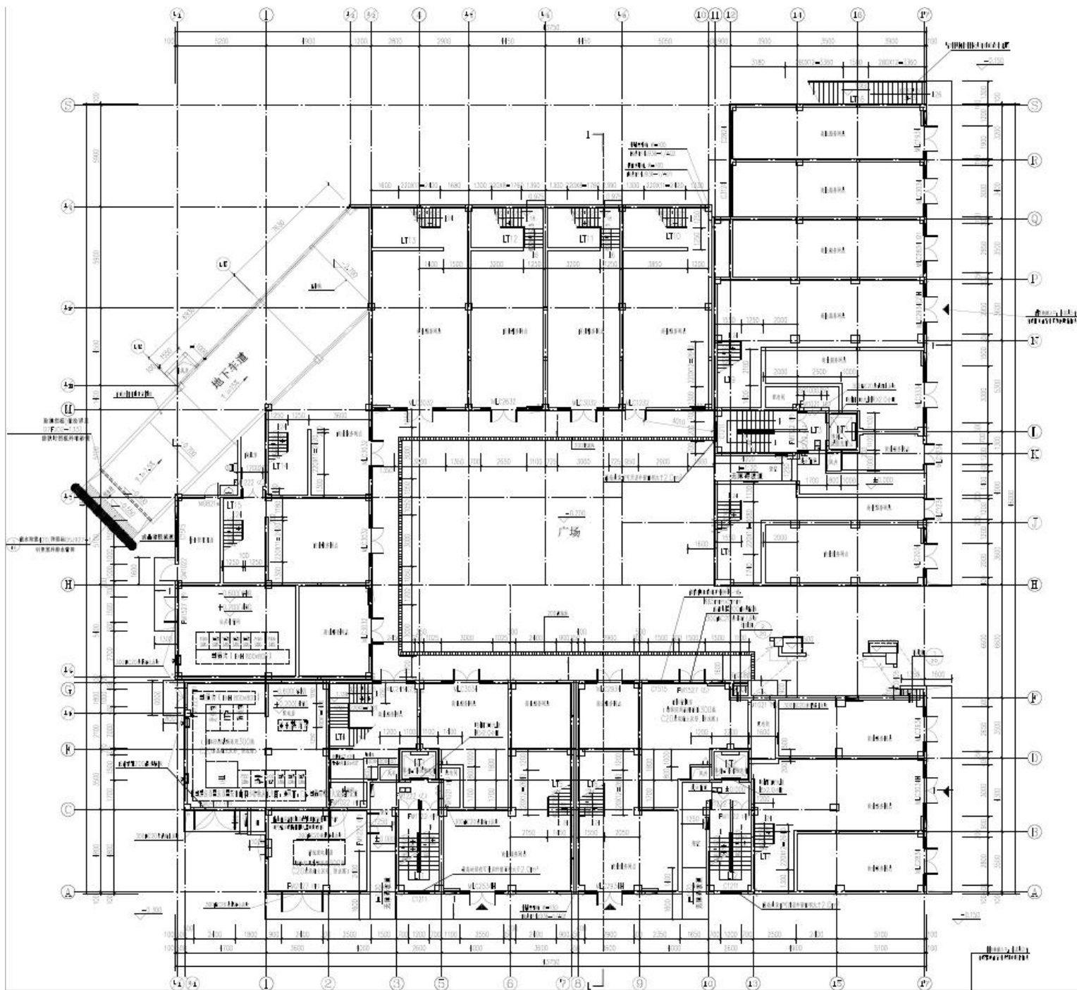
一层平面图 (变更前)
