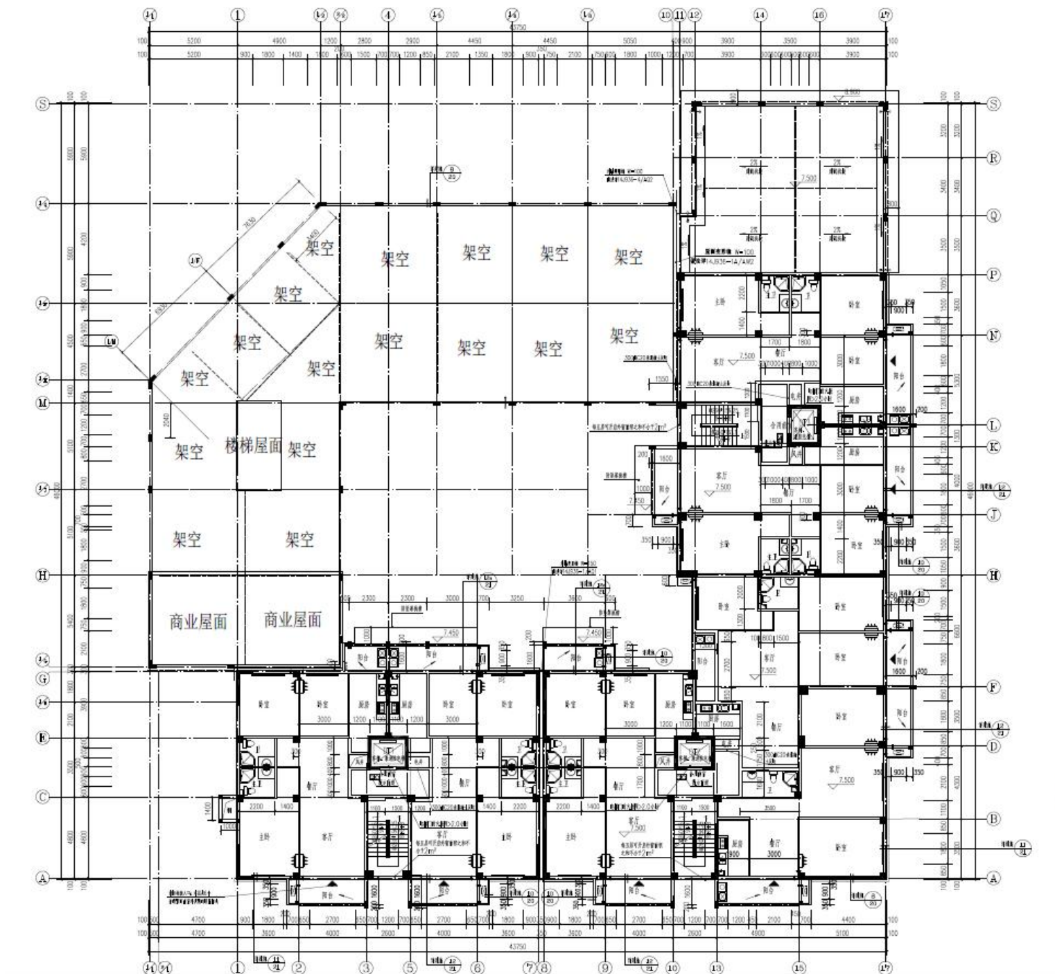
三层平面图（变更后）
