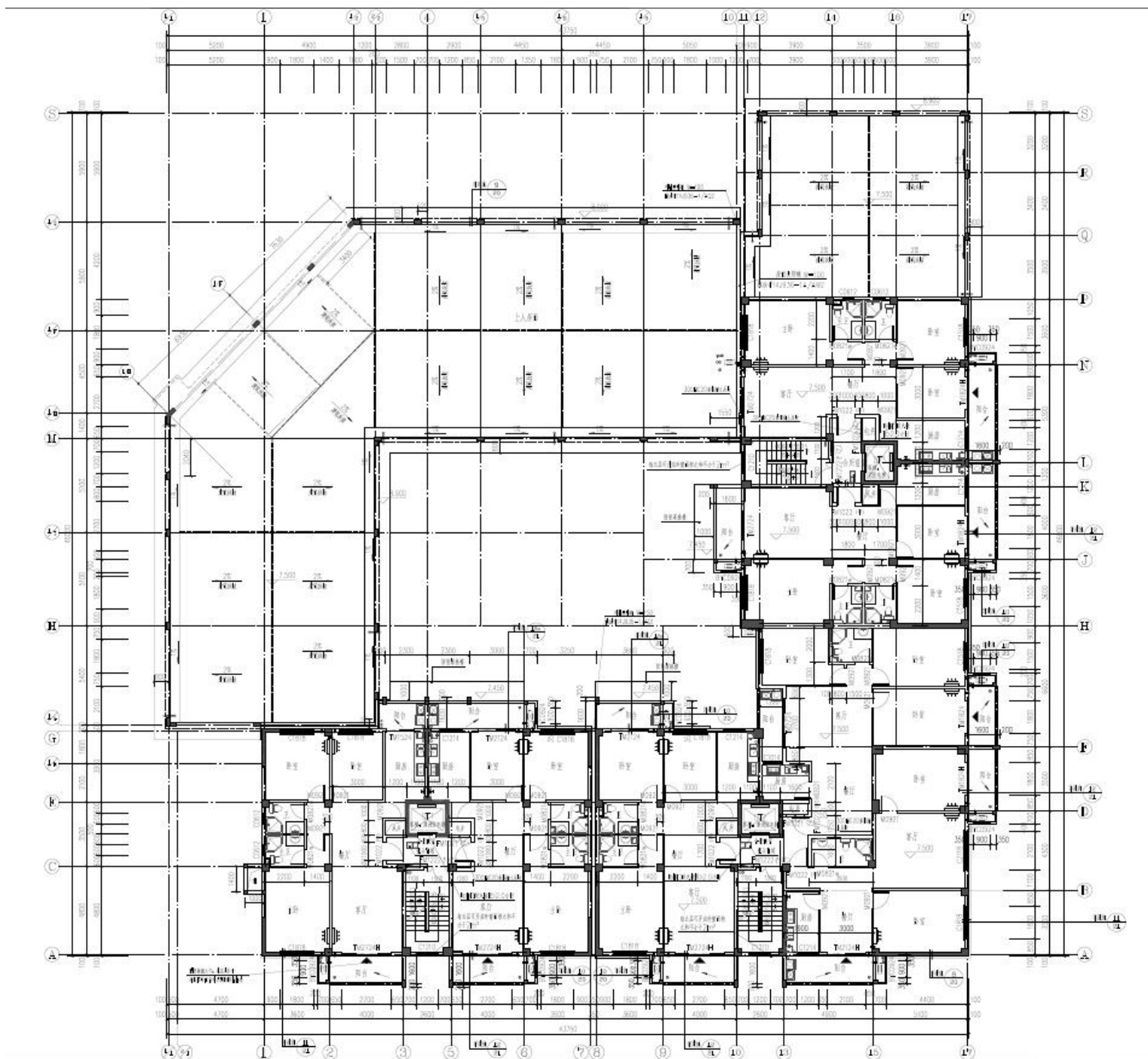
三层平面图（变更前）
