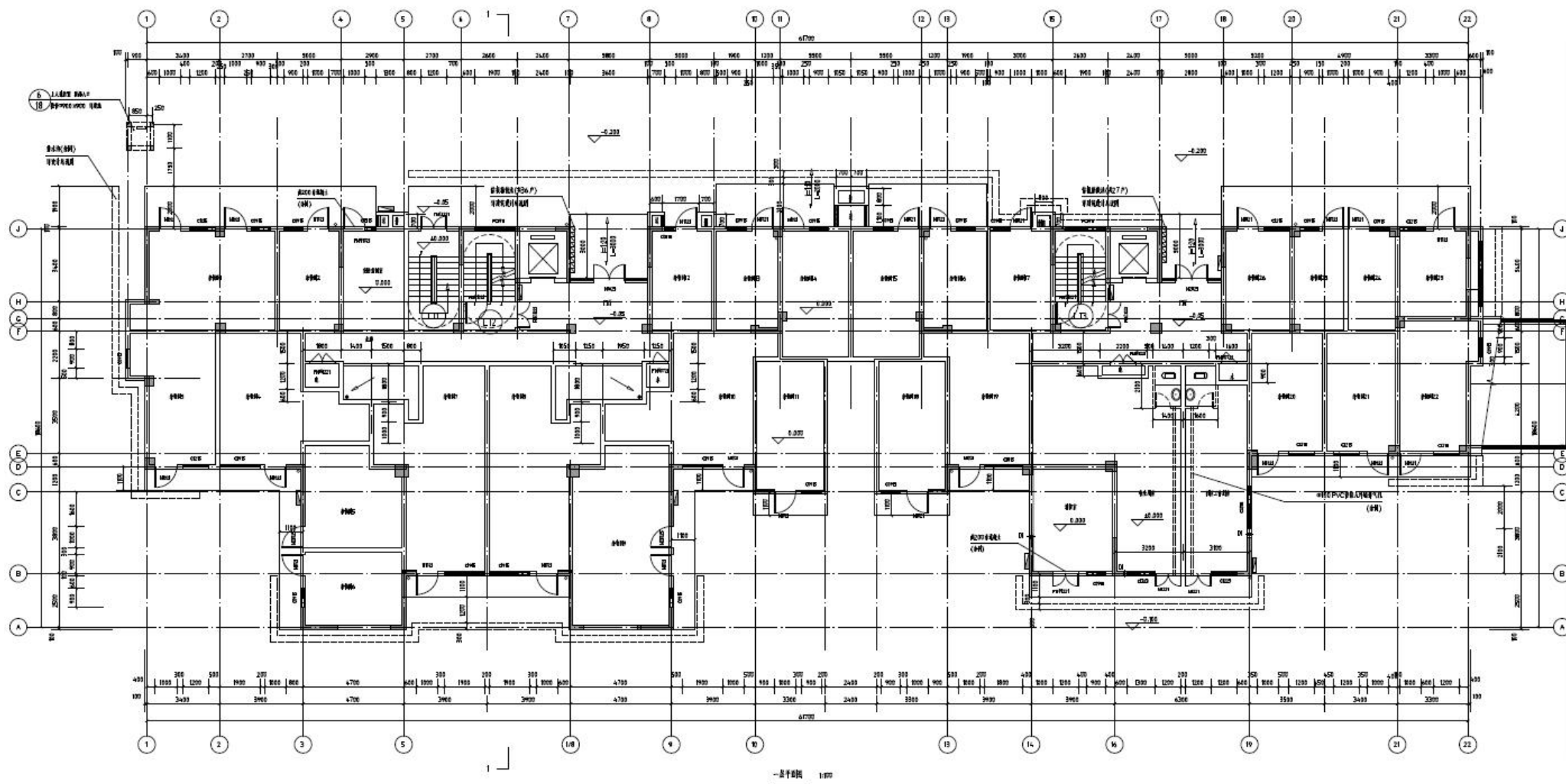
变更后一层平面图
