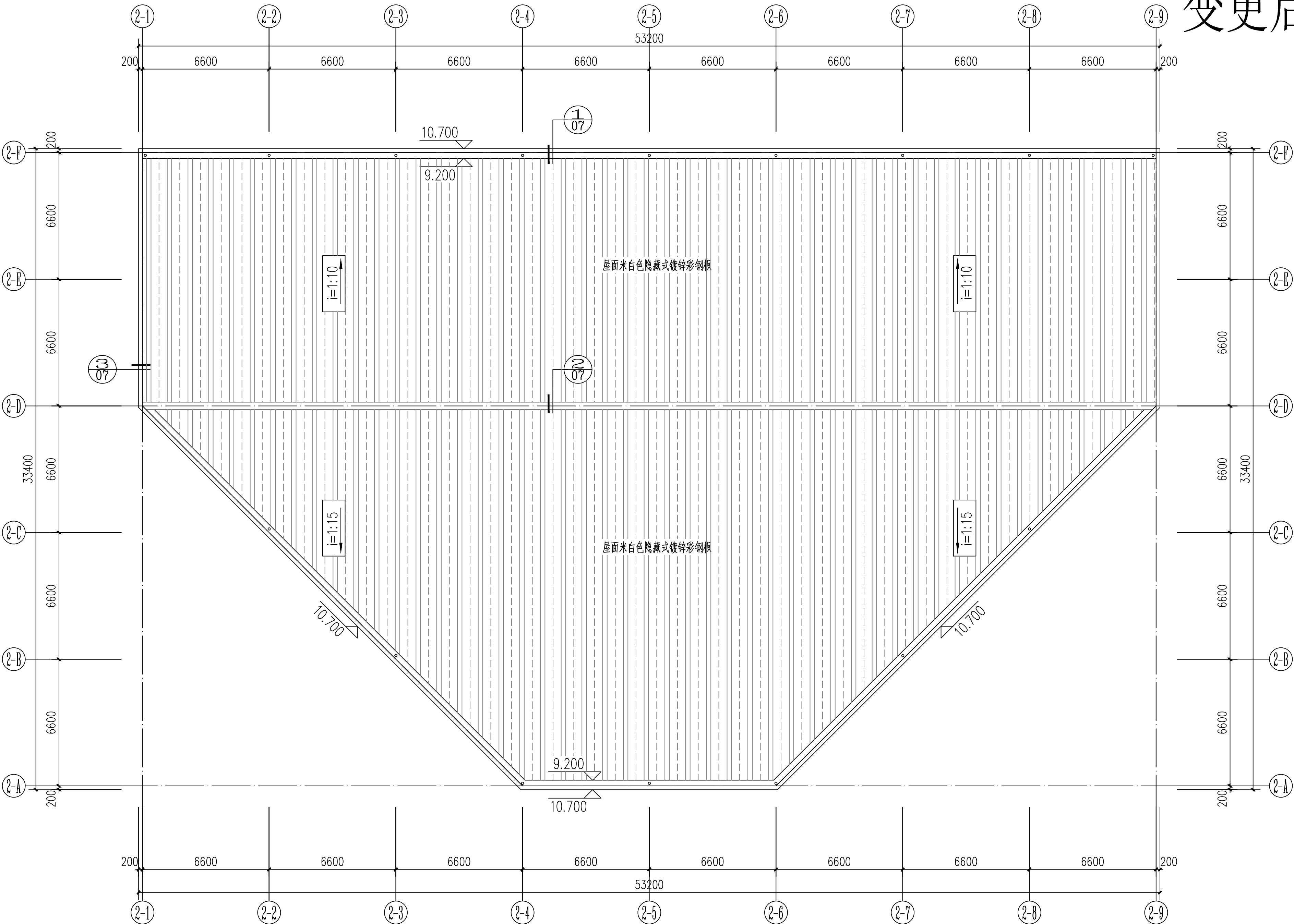
变更后屋面层平面图 1:150
