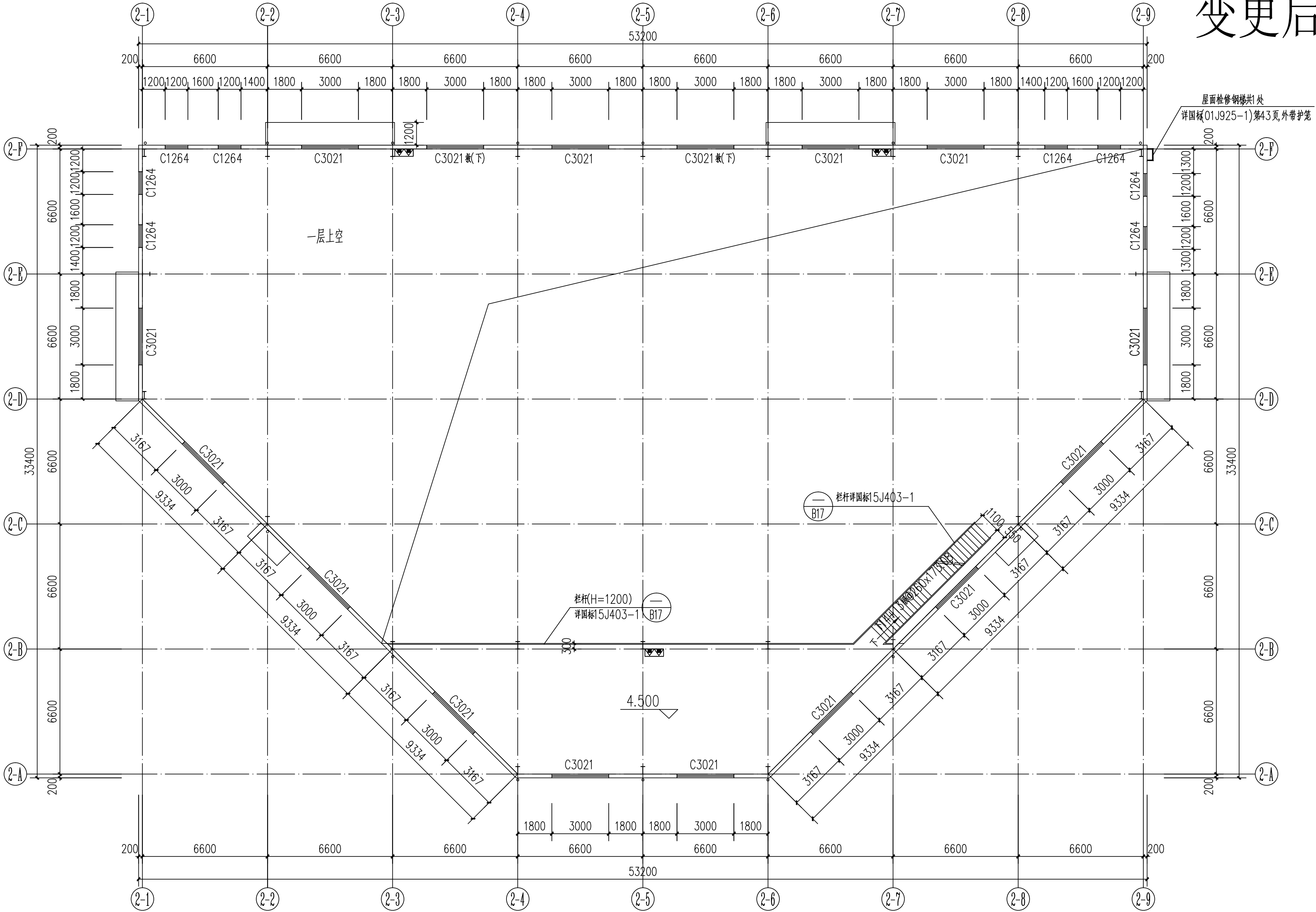
变更后二层平面图 1:150
