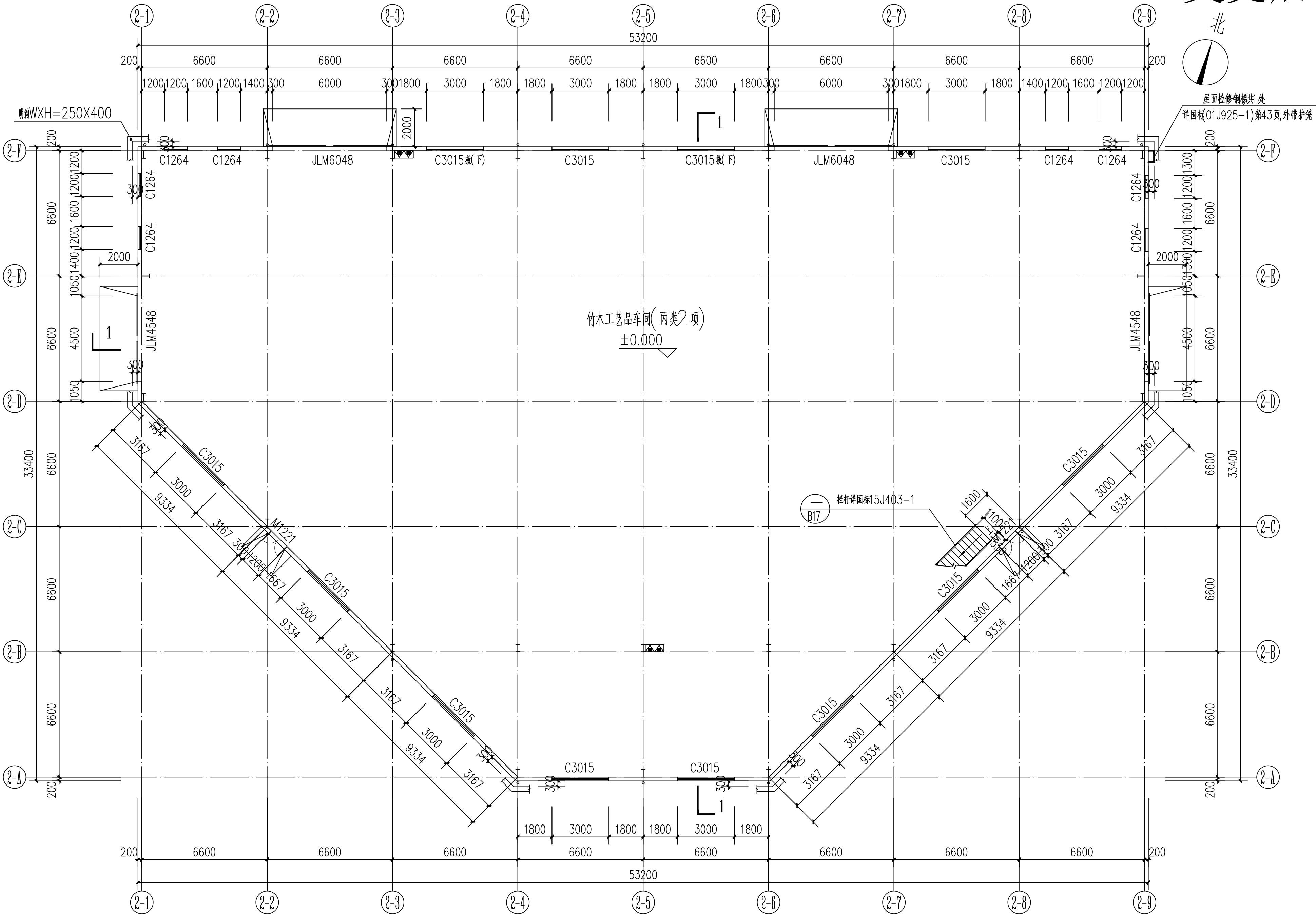
变更后一层平面图
