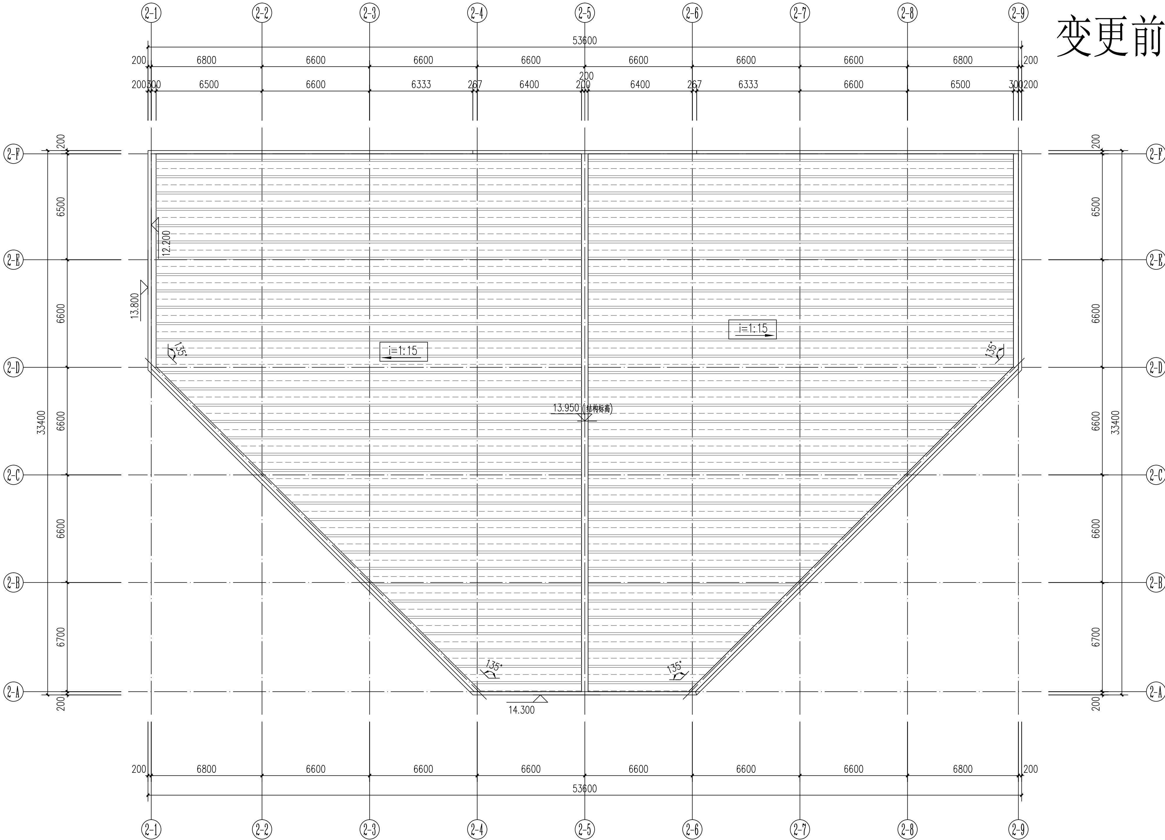
变更前屋面层平面图 1:150
