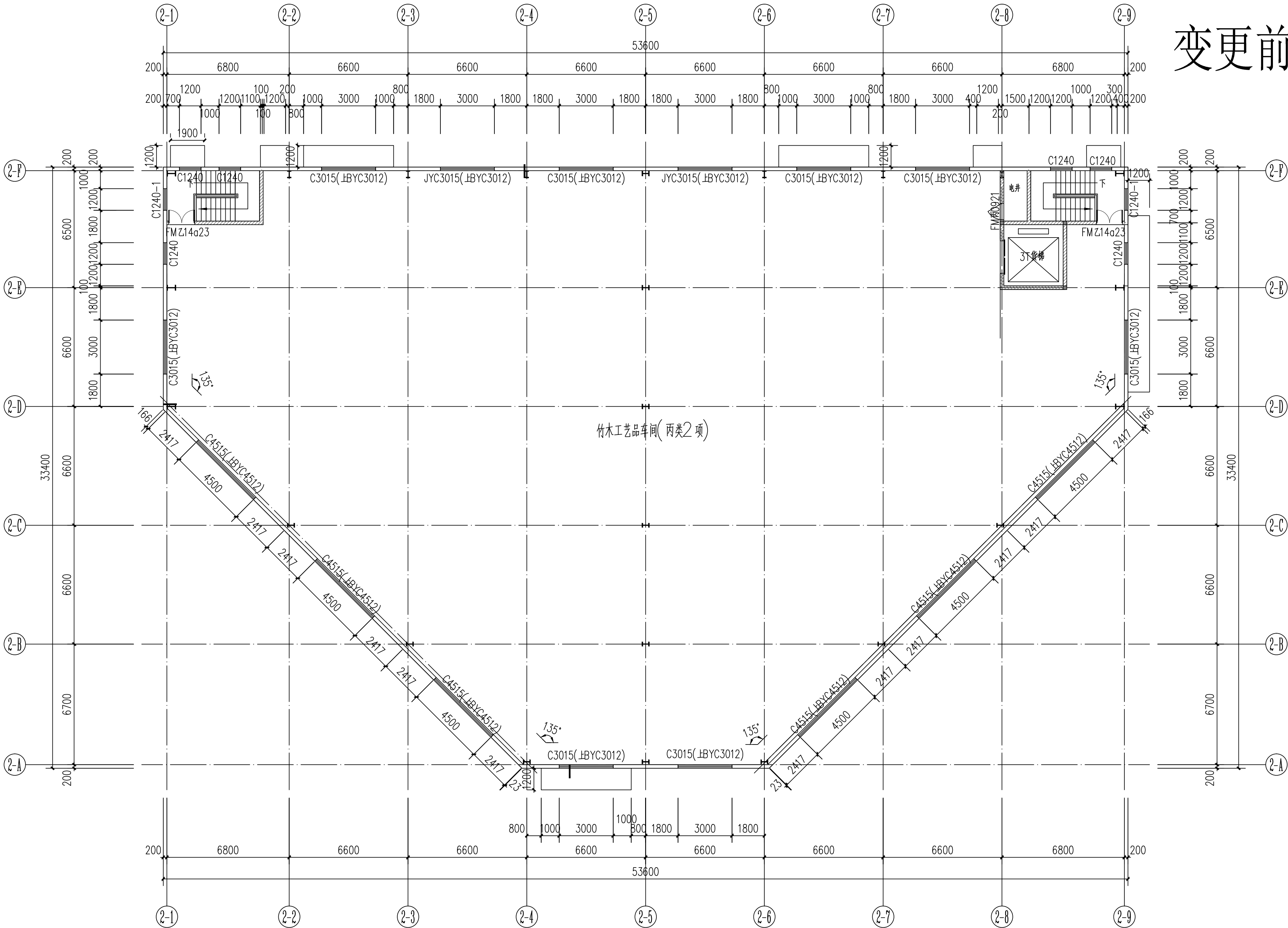
变更前二层平面图 1:150
