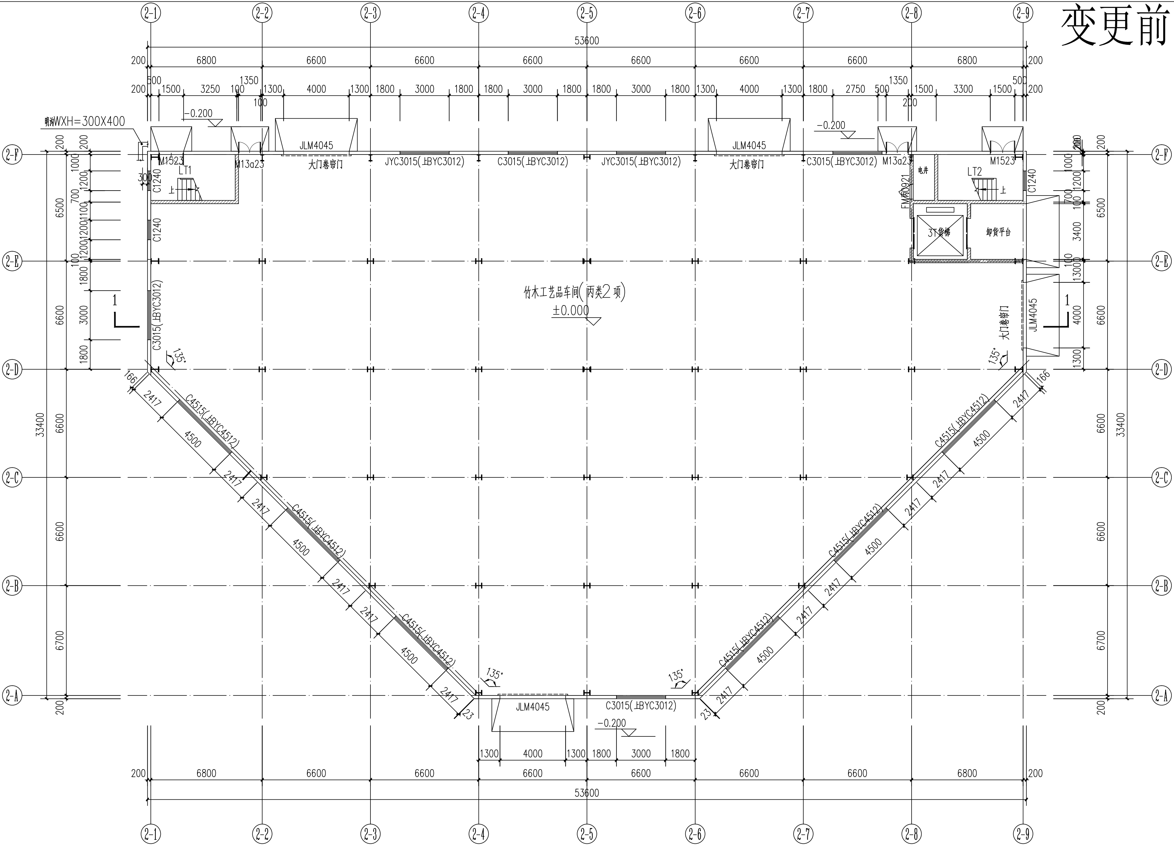
变更前一层平面图
