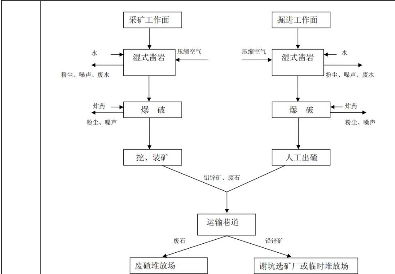
插图 3-5 谢坑矿段现有工程采矿工艺及产污环节图
