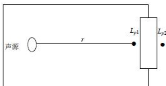
图 4.3-1 室内声源等效为室外声源图例
