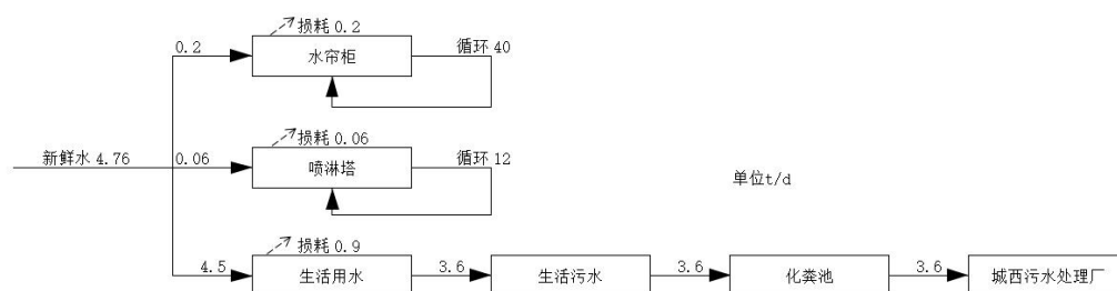
图 2.6-1 项目水平衡图 t/d
