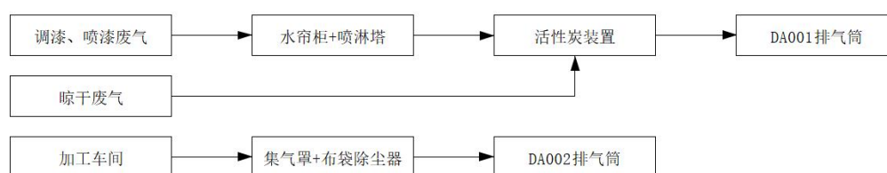
图 4.1-1 废气流程图
