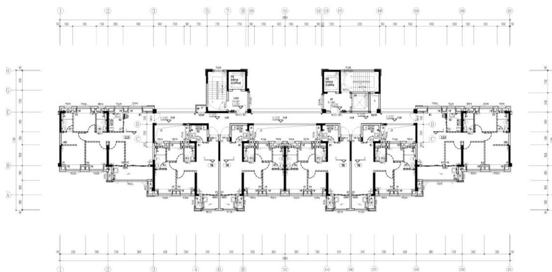
15、11#标准测平面图（原设计）
