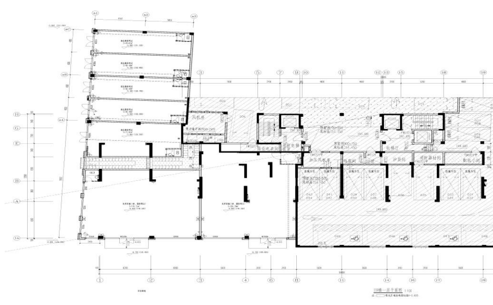
13、11#一层平面图（原设计）
