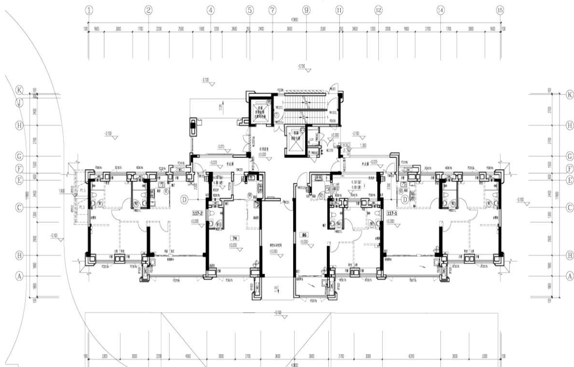
9、10#一层平面图（原设计）
