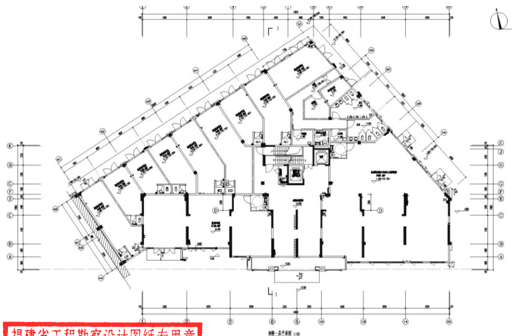
6、9#一层平面图（变更后）
