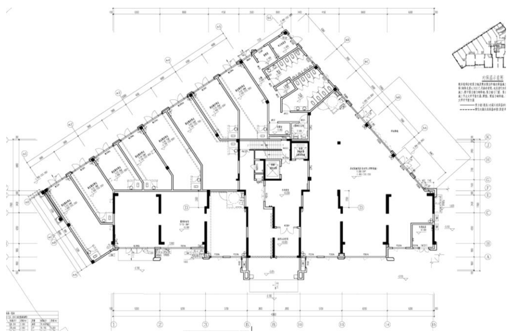
5、9#一层平面图（原设计）
